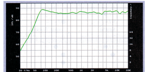
Quadral: Über das gesamte Spektrum vorbildlich glatter Verlauf, im Oberbass minimaler Anstieg.
