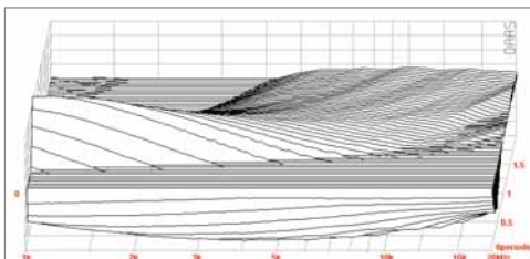
Abbildung 2: perfektes Ein- und Ausschwingen des AURUM Bändchens
