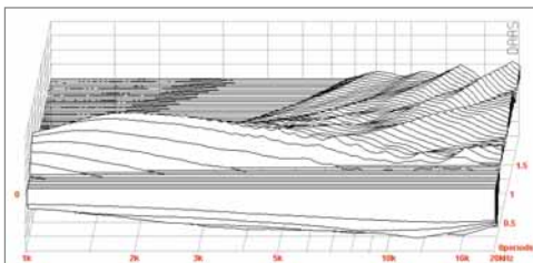
Abbildung 1: verzögertes Ein- und Ausschwingen einer konventionellen Metallkalotte
